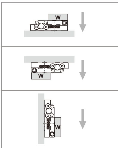
圖1 集中負載質量: W(kg)
