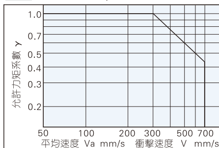
圖機2 允許力矩系數: γ
