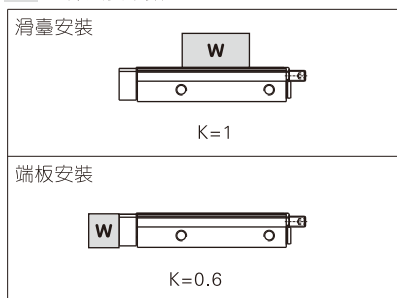
圖3 工件安裝系數: K
