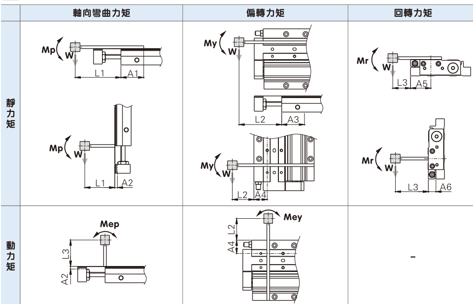
圖2 外伸量: Ln(mm)、力矩中心位置距離修正值: An(mm)
