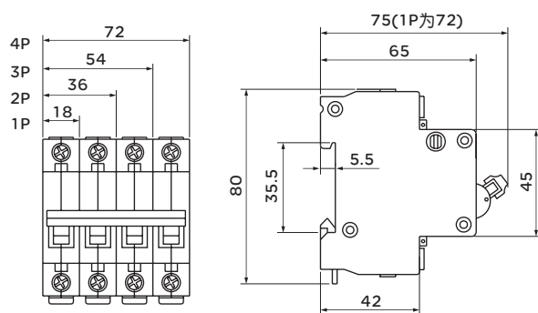
图4 外形尺寸与安装尺寸
