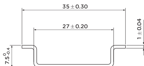
图5 安装轨尺寸
