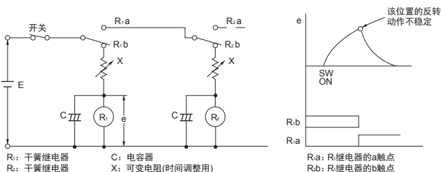
图1 按时间顺序使用干簧继电器使其工作的错误实例
