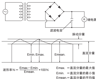
图3：直流线圈的输入电源
