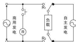
1) R_1, R_2 : R的触点 R : 2极形的继电器
