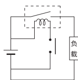
图4：线圈施加电压与电压降压
