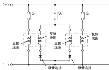
图3: 置位线圈、复位线圈的并联连接
