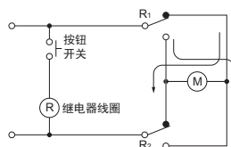
3) R_1, R_2 : R的触点 R : 2极形的继电器
