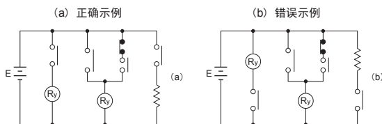
图1：负载与触点的连接
