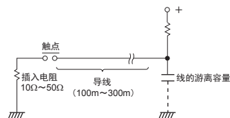
图4：等价电路
