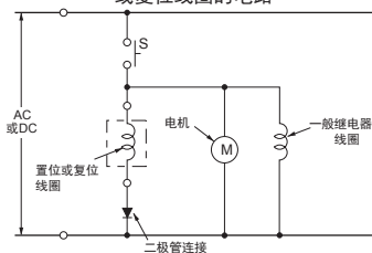
图4: 感性负载并联组入置位线圈或复位线圈的电路
