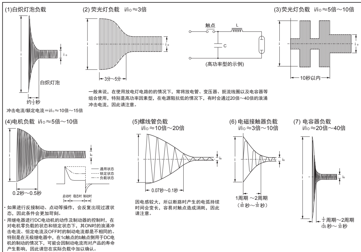
图3：负载的冲击电流波和时间的关系
