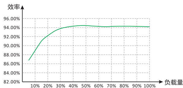
3C10-20K 效率曲线
