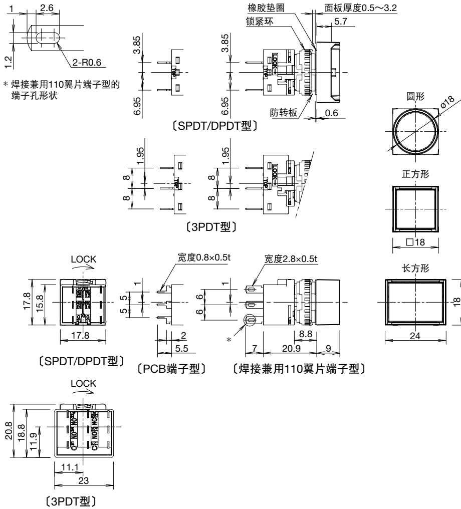
SPDT/DPDT 型 TOP
