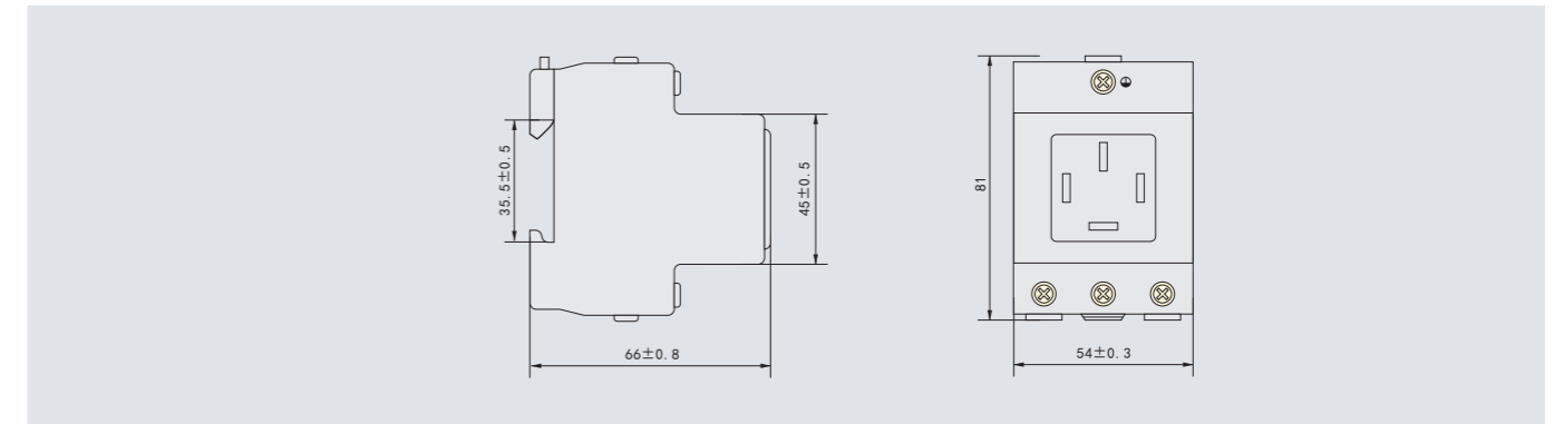
图 2、AC30-25/3D 440~外形及安装尺寸
