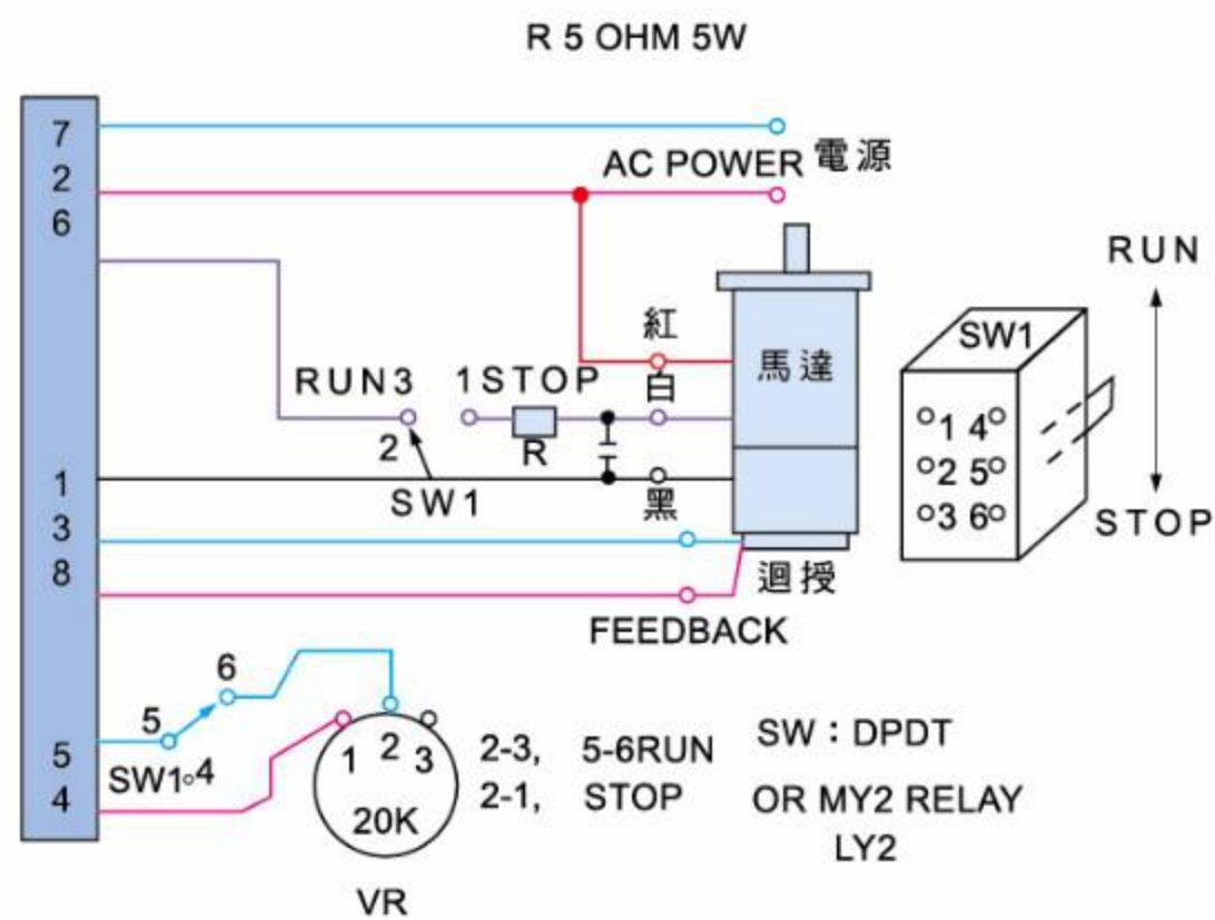
SS31 HR SS32 HR 配線圖
