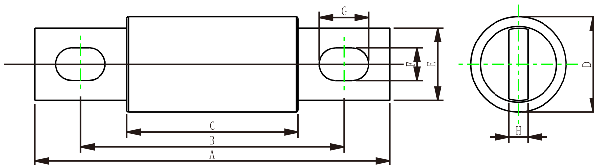
外形及安装尺寸(mm)
