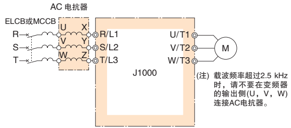
连接图
