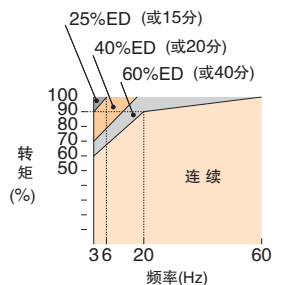
本公司标准电机的容许负载特性
