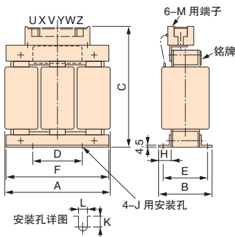
外形图 1
