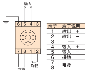
连接图
